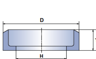
Чашечный круг, профиль 6F
