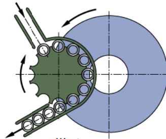
Шлифование напроход (подача вращением)
