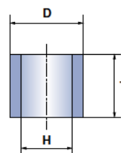
Кольцо, профиль 5420
