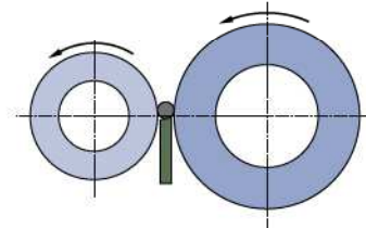
Шлифование напроход цилиндрических роликов
