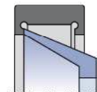
Шлифование борта наружного кольца
