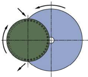
Двухстороннее шлифование, цилиндрические/конические ролики
