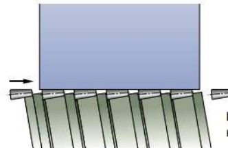
Шлифование напроход цилиндрических роликов
