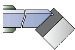
Шлифование дорожки и упорного борта внутреннего кольца
