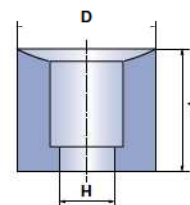
Чашечный круг, профиль 5ST
