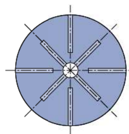
Шлифовальный круг, профиль 36ST
