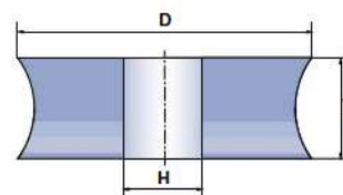
Шлифовальный круг, профиль 1-S
